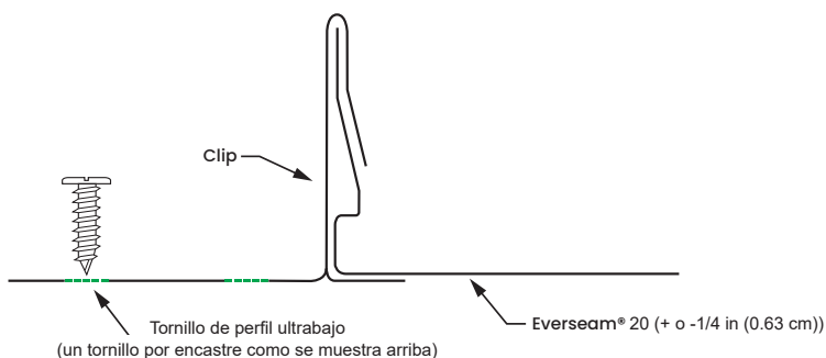
Sección transversal del panel colocado
